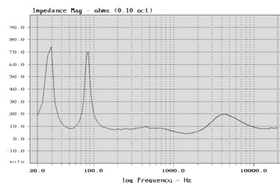
阻抗曲线
