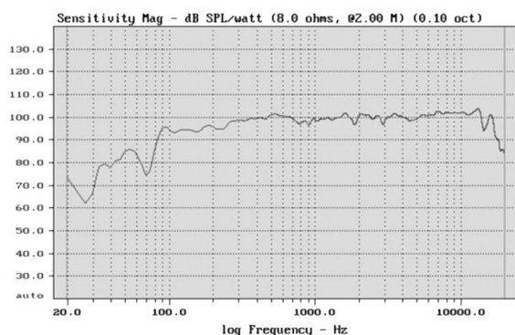
频响曲线
